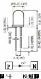
LED接腳圖
